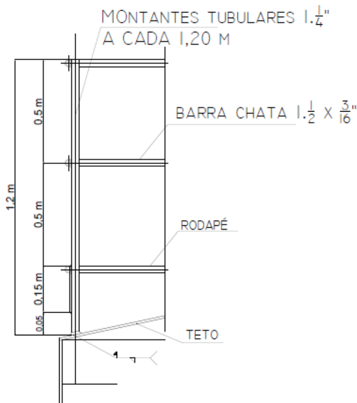
DETALHE GUARDA CORPO (TOPO DO RESERVATÓRIO)
