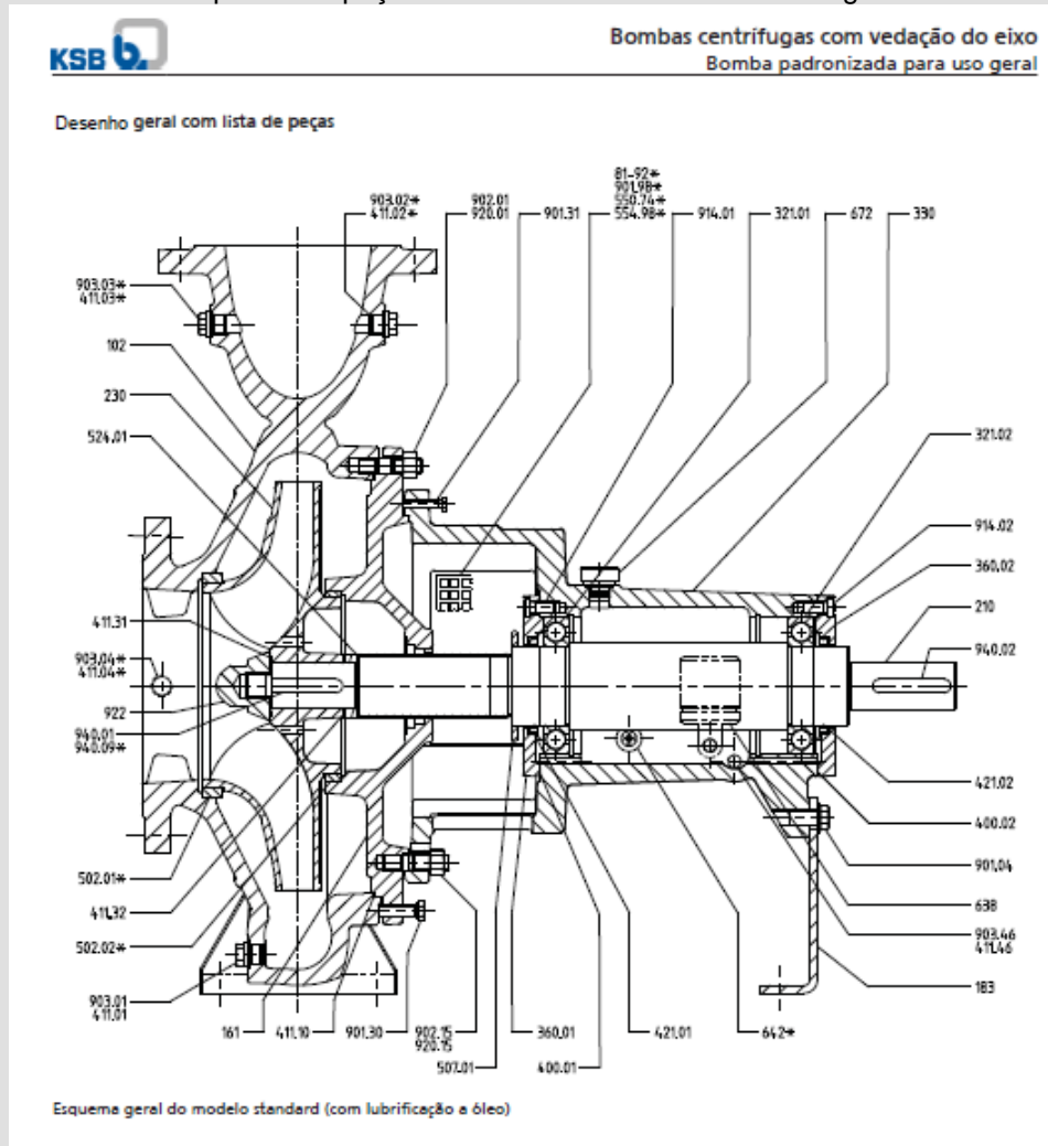
1A - Esquema de peças da bomba - Manual Técnico Meganorm N/2013:
